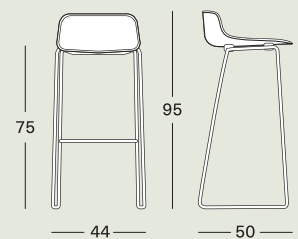
P 8370, U 8371 Sgabello alto slitta / Bar stool high sled base
