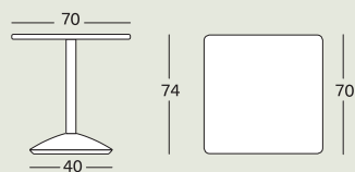
BA30 Tavolo quadrato Altezza 74 cm / Square table Height 74 cm
