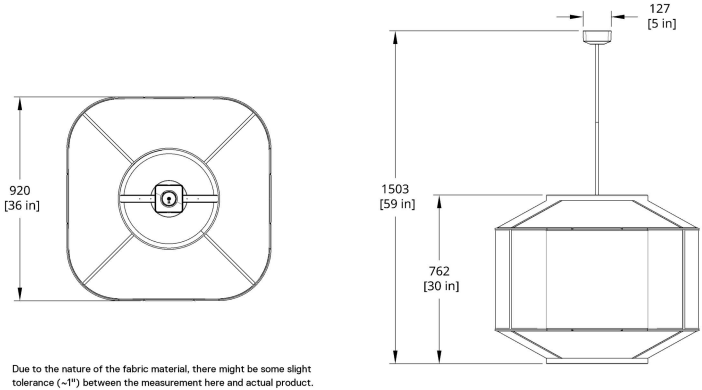
ALP-36-ST AllSew Pendant 36" Stem Dimension
