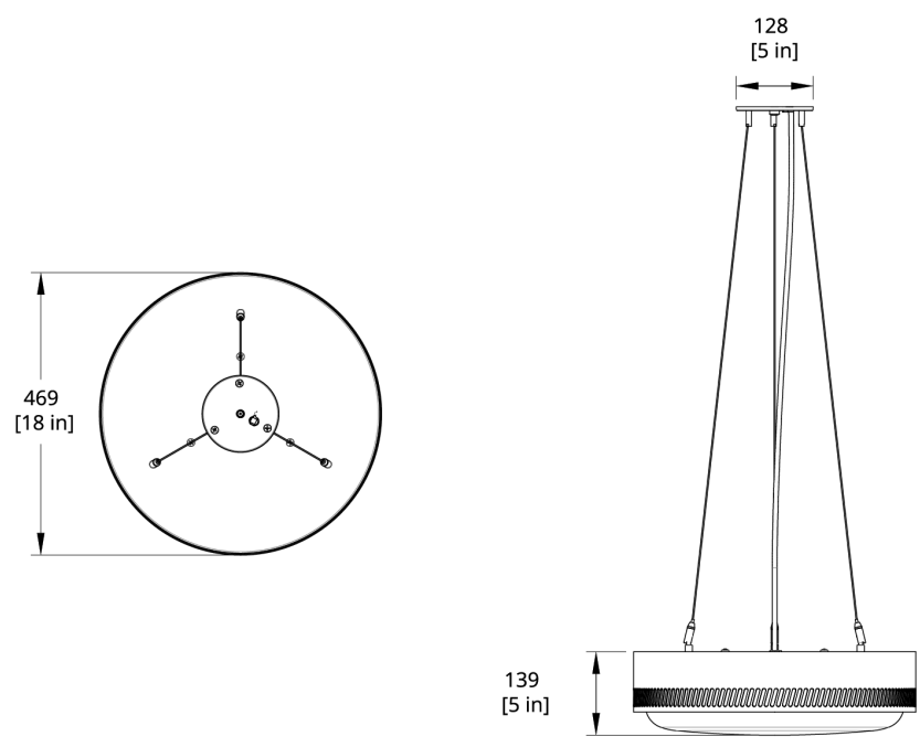
CTP-18 Centro Pendant Dimension
