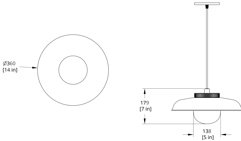
HP-8-B Hoist Pendant Large Diffuser Dimension
