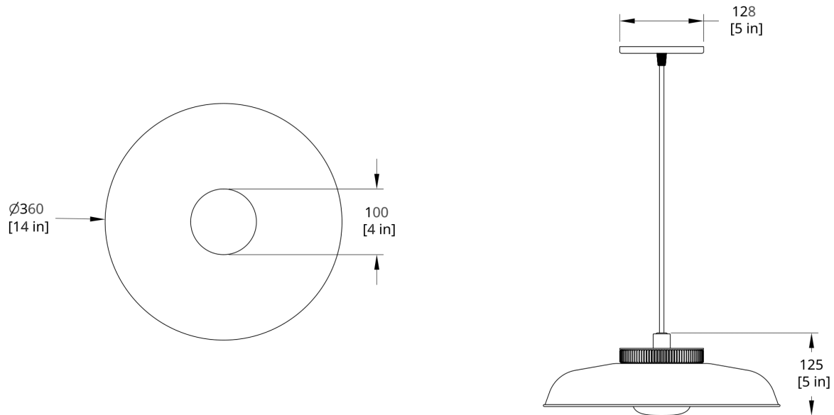
HP-14-A Hoist Pendant Small Diffuser Dimension
