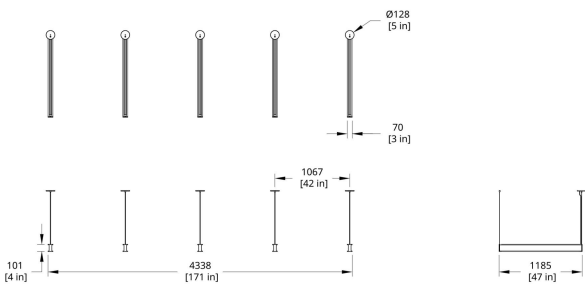
LS Latis Array 4' Dimension
