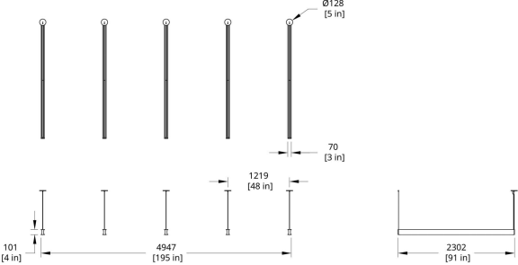
LS Latis Array 8' Dimension
